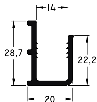
31 - Porta Blisan Inferior Peso: 0,38 Kg/m
