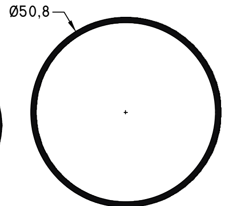
924 - Caño redondo de 50,8 mm e1,5 peso: 0,63 Kg/m
