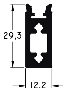
202 - Porta Hoja Largo std.: 6030 mm peso: 0,57 Kg/m
