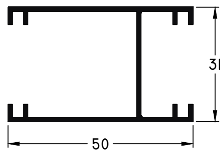
492 - Travesaño peso: 0,54 Kg/m
