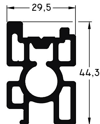
095 - Anclaje BBA aluminio peso: 1,34 Kg/m
