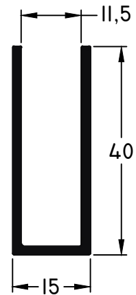
456 - U de 15 x 40 mm peso: 0,43 Kg/m
