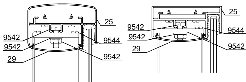
Opciones con pasamano recto
