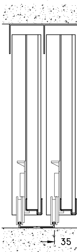
Detalle Vertical cantonera de 18mm.
