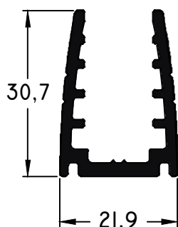
201 - Marco Largo std.: 6030 mm peso: 0,52 Kg/m
