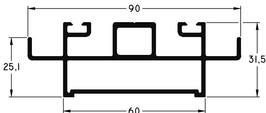
192 - Travesaño de Techo peso: 1,27 Kg/m
