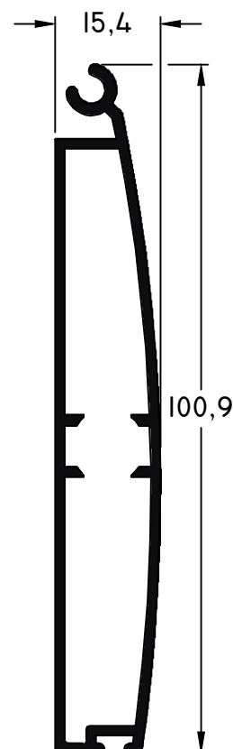
626 - Zócalo peso: 0,90 Kg/m
