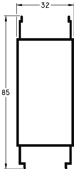
415 - Revestimiento Tubular peso: 0,75 Kg/m
