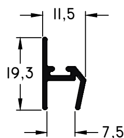
438 - Cierre vidrio 180° peso: 0,15 Kg/m
