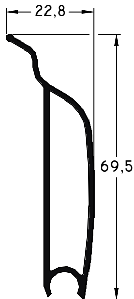
627 - Tablilla de Comando peso: 0,49 Kg/m
