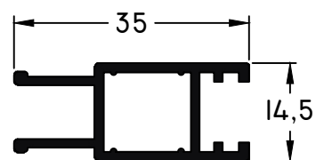
944 - Hoja de Mampara peso: 0,35 Kg/m
