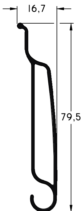
983 - Primera tablilla cortina regulable c/felpa peso: 0,52Kg/m
