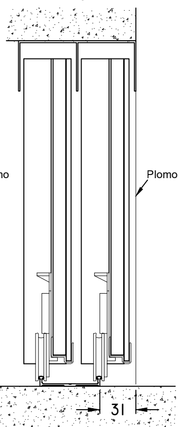
Detalle Vertical cantonera de 15mm.
