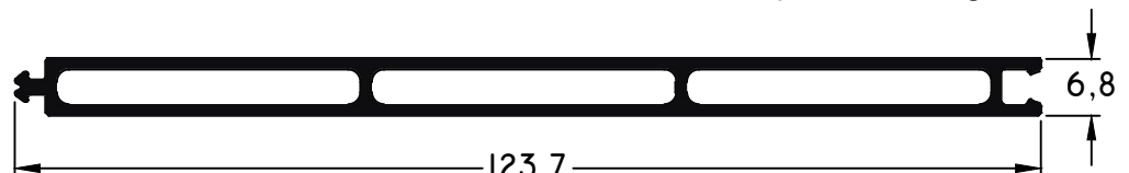
398 - Revestimiento Tubular peso: 0,91 Kg/m
