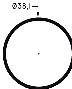
996 - Caño Redondo de 38,1 mm e1,5 peso: 0,47 Kg/m
