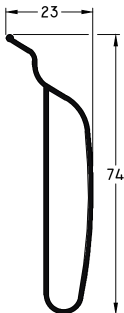
628 - Tablilla Tubular peso: 0,48 Kg/m
