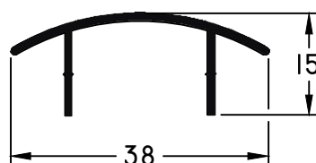
494 - Tapa peso: 0,19 Kg/m
