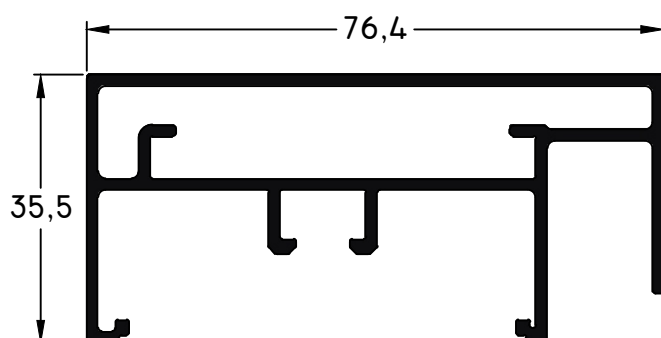
032 - Pasamanos Recto 35,5 mm peso: 1,15 Kg/m
