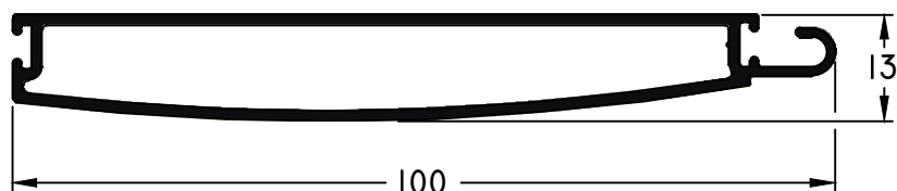
624 - Zócalo Cortina Común
