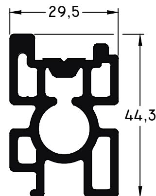
095 - Anclaje BBA aluminio peso: 1,34 Kg/m
