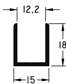
469 - U 15 x 18 mm peso: 0,18 Kg/m
