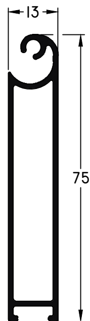
984 - Zócalo cortina regulable c/felpa peso: 0,67 Kg/m
