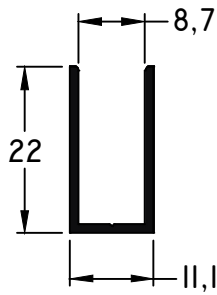
466 - U 11,1 x 22 mm peso: 0,17 Kg/m
