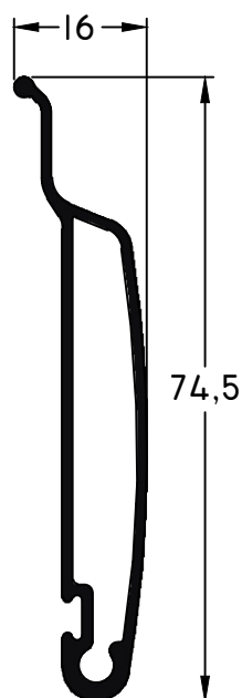
899 - Cortina regulable c/felpa peso: 0,53 Kg/m
