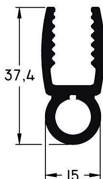
203 - Hoja Largo std.: 6030 mm peso: 0,64 Kg/m
