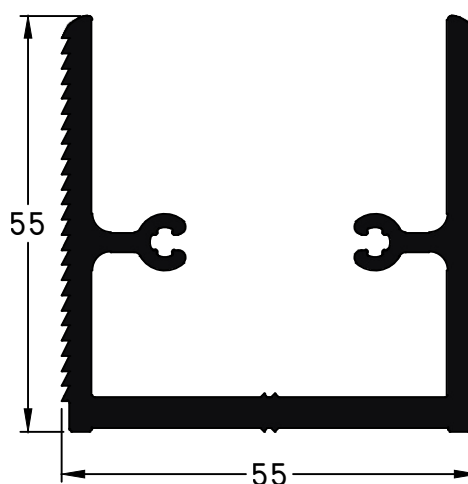
47 - U Armado FI peso: 1,77 Kg/m
