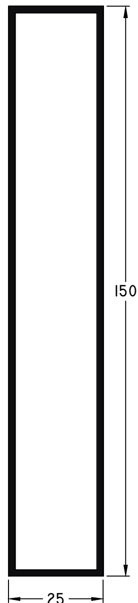
472 - Tubo 150 x 25 mm e: 1,7 peso: 1,58 Kg/m
